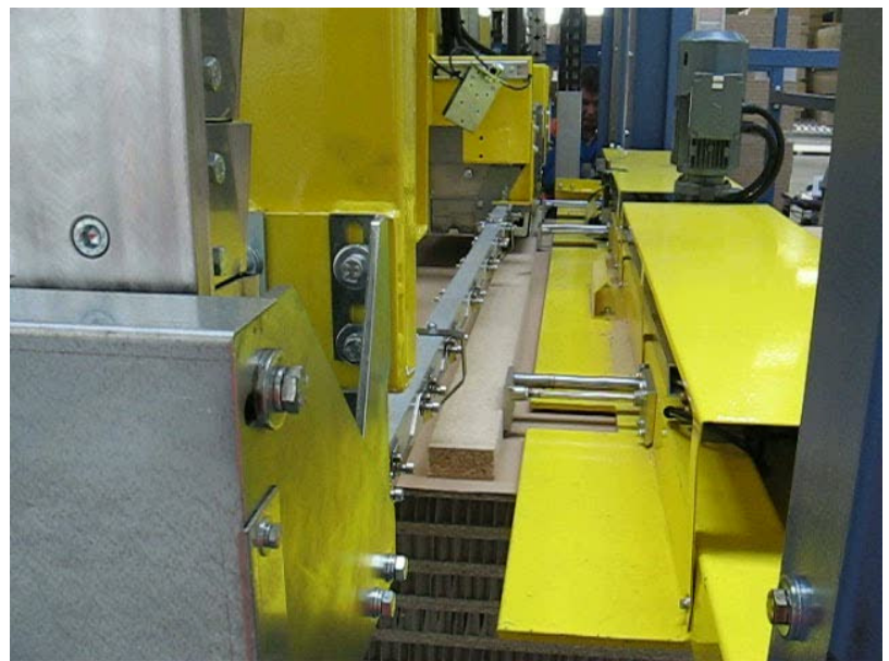
Übergabe der Leisten vom vertikalen Leistentransport in die Umreifungsposition
